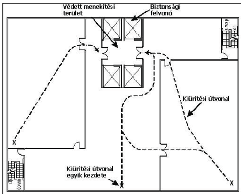
5. Biztonsági felvonó előterében kialakított átmeneti menekülési terület
