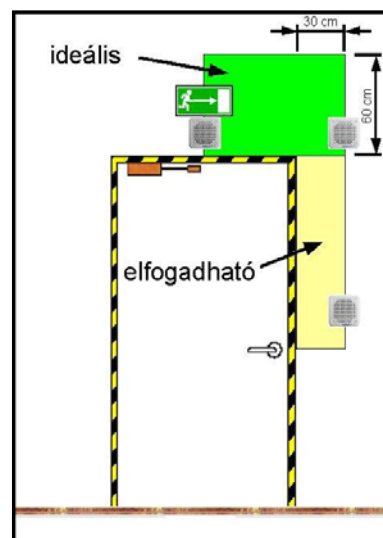
7. ... és elhelyezése egyszárnyú ajtó
