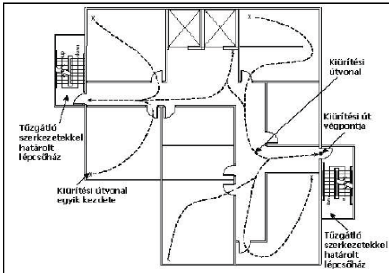
4. A kiürítési útvonal a legtávolabbi pontokról indul és a biztonságba vezető kijáratoknál végződik
