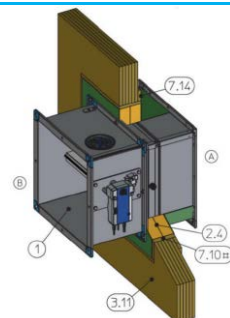
3D5.6.7. ábra. Tűzgátló csappantyú száraz (lágylezárásos) beépítése CLT fal síkján belül
