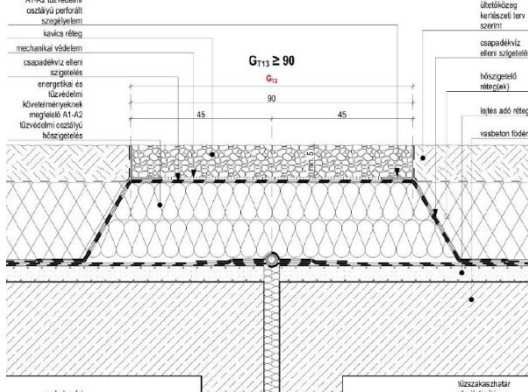
3F6 sz. ábra: extenzív zöldtető tetősíkbán tartott tetőszinti tűzterjedés elleni gátja kialakításának példája
