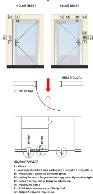
G20. ábra: Egyszárnyú, elektromos zárással rendelkező homlokzati ajtók / tűzgátló vagy légpótló ajtók – „D” típus
