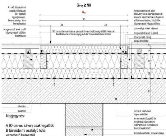
3F5 sz. ábra: magastető tetősíkbán tartott tetőszinti tűzterjedés elleni gátja kialakításának példája, vasbeton koporsófödém esetén
