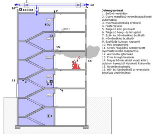
H-4. ábra: Példa túlnyomásos füstmentes lépcsőház tetősínti frisslevegő beszívásának lehetőségére
