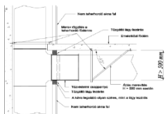
D5.3.5. ábra. Nem teherhordó aknafalu épített nagy méretű csappantyú a földéhez és az akna teherhordó falához mereven rögzített légesatornákkal
