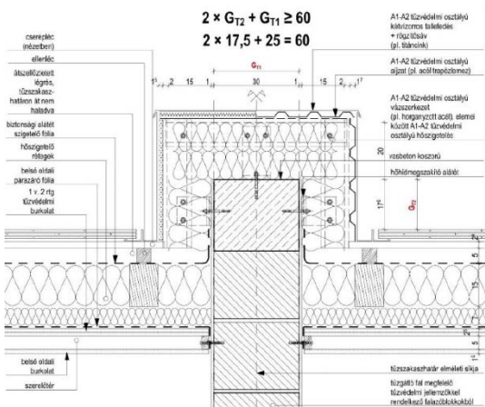
3F3 sz. ábra: magastető tetősíkból kiemelkedő tetőszinti tűzterjedés elleni gátjának példája
