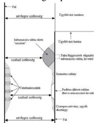
C4. ábra: Közlekedési úton 1,90 m-nél alacsonyabban elhelyezett berendezési tárgyak szabad szélességére való hatása
