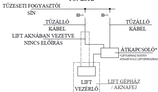
(B) LIFT VEZÉRLŐ EGY KÁBELT TUD FOGADNI!
