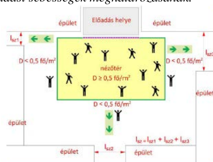
7. ábra: A kezdeti szabad menekülési szélesség zöld vonallal, a menekülésre figyelembe vett útvonalak legkisebb szabad szélességeinek összege piros méretnyilakkal szemléltetve (a második számítási metódushoz kapcsolódó ábra)
