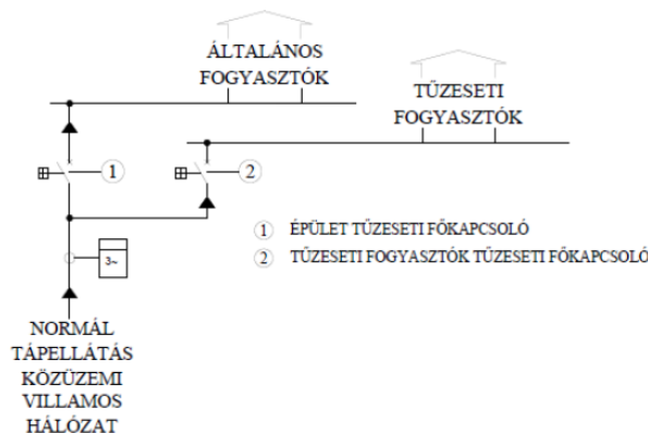
5. ábra Tüzeseti fogyasztók általános ellátása
