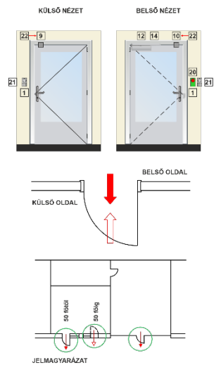
G18. ábra: Egyszárnyú, elektromos zárassal rendelkező homlokzati ajtók / tűzgátló ajtók – „B” típus
