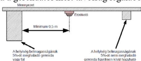
3. ábra Füstérzékelő távolsága gerendáktól
