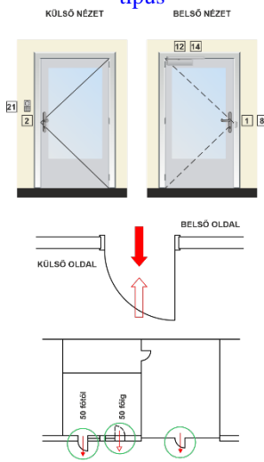
G17. ábra: Egyszárnyú, elektromos zárassal rendelkező homlokzati ajtók / légpótló ajtók – „A” típus
