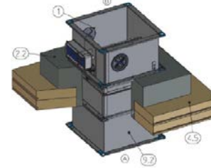
3D5.6.3. ábra. Tűzajtó csappantyú beépítése vasbeton gallerba CLT földem síkjára
