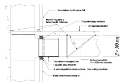
D5.3.5. ábra. Nem teherhordó aknafalú épített nagy méretű csappantyú a földéhez és az akna teherhordó falához mereven rögzített légesatornákkal
