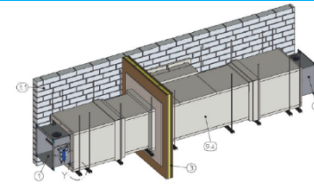
3D5.5.3. ábra. Tűzajtó csappantyú beépítése külön függesztéssel a tűzszakaszhatár(ok) síkjától távol
