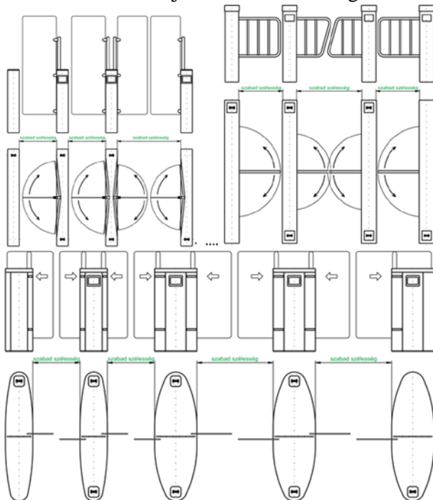
C8. ábra: Ajtók szabad szélessége
