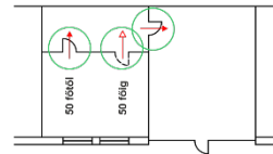
G2. ábra: Egyszárnyú, zárás nélküli belső ajtók / tűzgátló ajtók – „B” típus
