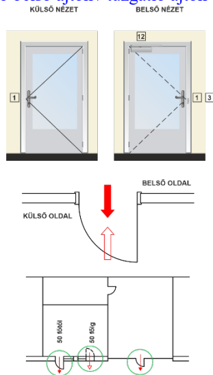
G9. ábra: Egyszárnyú, elektromos zárással rendelkező belső ajtók / tűzgátló ajtók – „C” típus
