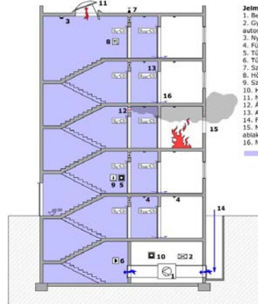
H-2. ábra: Példa előteres túlnyomásos füstmentes lépcsőház kialakítására, szabályozott üzemi ventilátorral, túlnyomás levezető kupolával
