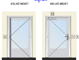
G13. ábra: Egyszárnyú, mechanikai zárással rendelkező homlokzati ajtók / tűzgátló ajtók – „A” típus
