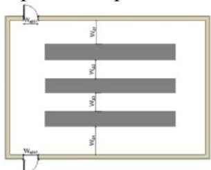
C7. ábra: l_{sz} = \sum l_{út} illetve \sum l_{ajtó} közül a kisebbik értékkel
