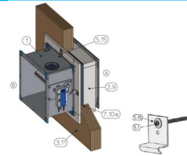
3D5.6.8. ábra. Tűzgátló csappantyú beépítése beépítő készlettel CLT fal síkján belül
