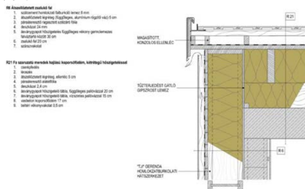
E3 sz. ábra. Falazott, átszellőztetett légréses homlokzatburkolattal ellátott fal és átszellőztetett légréses magastető csatlakozása
