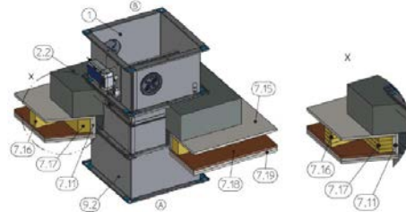
3D5.6.2. ábra. Tűzajtó csappantyú beépítése vasbeton gallerba egy fagerendás földem síkjára
