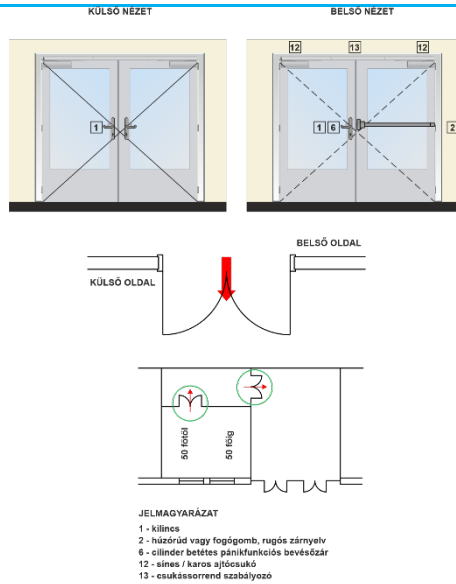
G25. ábra: Kétszárnyú, mechanikai zárral rendelkező belső ajtók / tűzgátló ajtók – „B” típus
