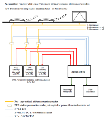
K.1.1-1. ábra: Automatikus (tűzjelző érzékelő általi) vésznyitás megoldásának példája
