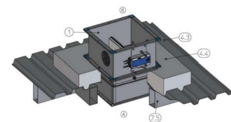
3D5.6.4. ábra. Tűzajtó csappantyú beépítése vasbeton gallerba könnyűszerkezetes földem síkjára
