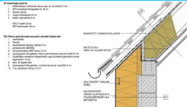
E2 sz. ábra. Falazott, éghető hőszigeteléssel ellátott fal és átszellőztetett légréses magastető csatlakozása
