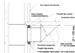
2D5.3.3. ábra. Nem teherhordó aknafalban épített, a födémhez mereven rögzített nagy méretű tűzvédelmi csappantyú
