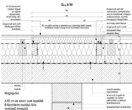
3F5 sz. ábra: magastető tetősíkból tartott tetőszinti tűzterjedés elleni gátja kialakításának példája, vasbeton koporsófödém esetén
