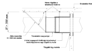
3D5.5.2. ábra. Nagyméretű csappantyú beépítése merev rögzítéssel tűzszakaszhatáron kívül
