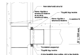
2D5.3.4. ábra. Nem teherhordó aknafalban épített kis méretű tűzvédelmi csappantyú a födémhez és az akna teherhordó falához mereven rögzített légcsatornákkal
