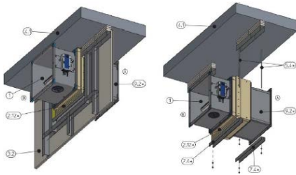
3D5.6.5. ábra. Tűzgátló csappantyú beépítése csúszó földémkapcsolattal és csappantyúbeépítő készlettel
