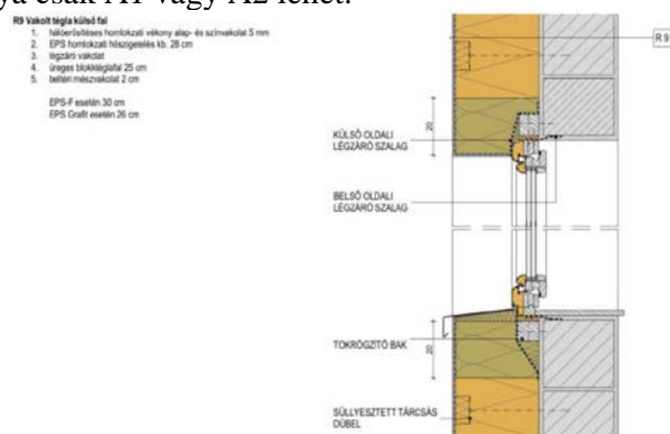
E5 sz. ábra. Falazott, vakolt homlokzati hőszigetelő rendszerrel ellátott fal ablakcsatlakozása E3.5. Az E5 sz. ábrán látható részletrajzon bemutatott megoldások tűzvédelmi vonatkozásai:
