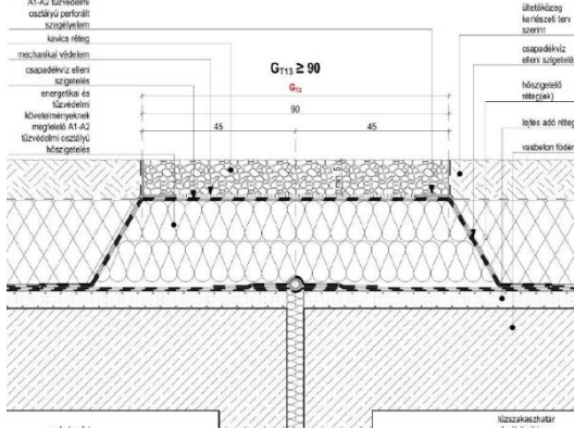
3F6 sz. ábra: extenzív zöldtető tetősíkból tartott tetőszinti tűzterjedés elleni gátja kialakításának példája
