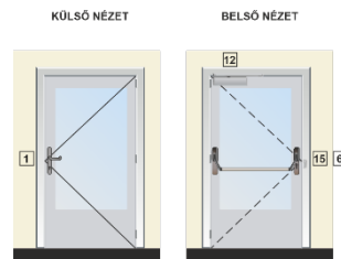
G14. ábra: Egyszárnyú, mechanikai zárással rendelkező homlokzati ajtók – „B” típus
