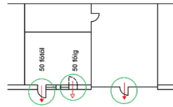
G13. ábra: Egyszárnyú, mechanikai zárással rendelkező homlokzati ajtók / tűzgátló ajtók – „A” típus
