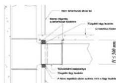
2D5.3.2. ábra. Nem teherhordó aknafalban épített, a födémhez mereven rögzített kis méretű tűzvédelmi csappantyú
