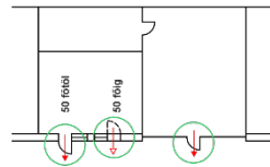
G15. ábra: Egyszárnyú, mechanikai zárással rendelkező homlokzati ajtók / tűzgátló ajtók – „C” típus
