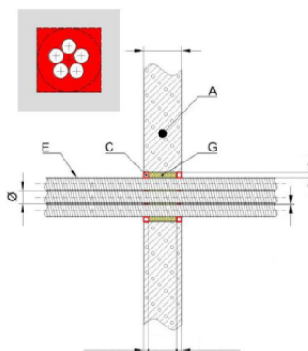
D1.1.3.2. ábra tűzvédelmi kitt lágy lezárásban (falátvezetés)
