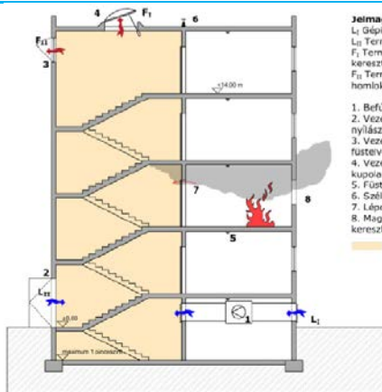
H-1. ábra: Példa a természetes hő- és füstelvezetéssel ellátott lépcsőház kialakítására különböző légpótlási variációkkal
