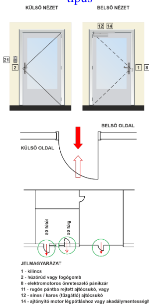
G19. ábra: Egyszárnyú, elektromos zárassal rendelkező homlokzati ajtók / légpótló ajtók – „C” típus
