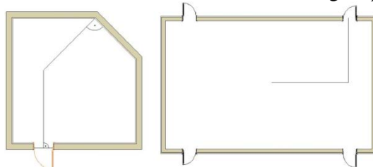
C2. ábra: Példák a kiürítési út hosszának megállapításáról
