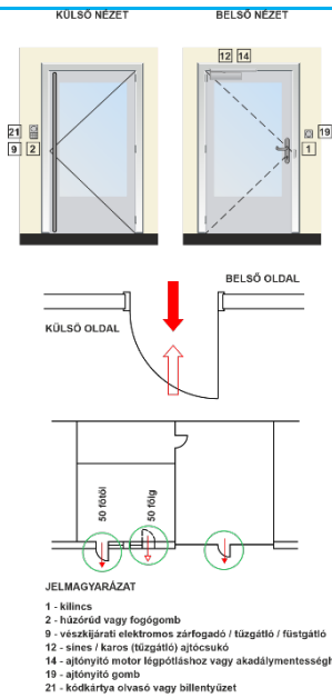
G17. ábra: Egyszárnyú, elektromos zárassal rendelkező homlokzati ajtók / légpótló ajtók – „A” típus
