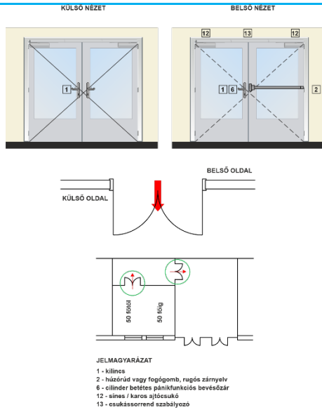
G25. ábra: Kétszárnyú, mechanikai zárassal rendelkező belső ajtók / tűzgátló ajtók – „B” típus
