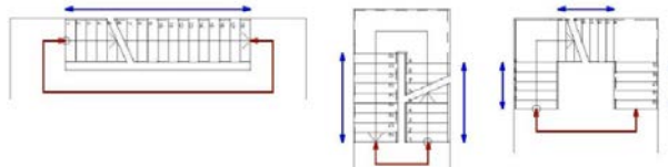
2A ábra: 2Lépcsőkarok és lépcsőkarok közötti útvonal hosszak
