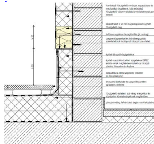
M2 ábra Terasztető lábazati csomópontjának elvi kialakítása
