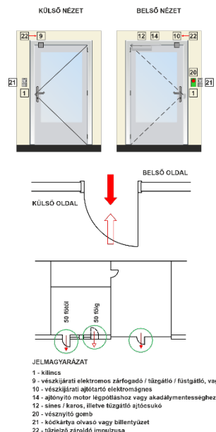
G20. ábra: Egyszárnyú, elektromos zárassal rendelkező homlokzati ajtók / tűzgátló vagy légpótló ajtók – „D” típus
