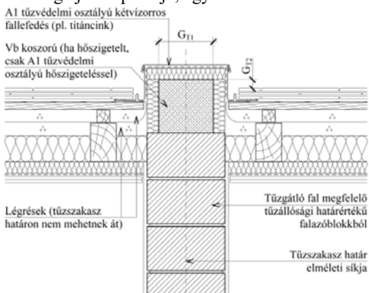
F1 sz. ábra: lapostető tetőszinti tűzterjedés elleni gátjának példája, egyszeres tűzfal
