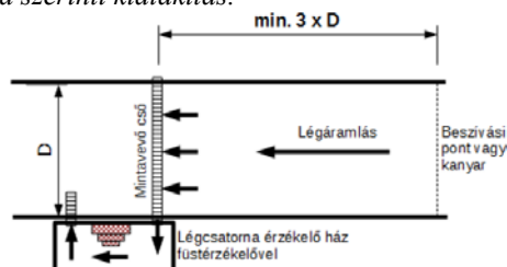
7. ábra Légtcsatorna érzékelő elhelyezkedése
