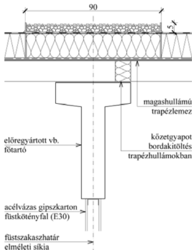
F5 sz. ábra: előregyártott vasbeton vázszerkezetű és könnyű tetőfödém térelhatároló szerkezetű épület tűzszakaszhatárához kapcsolódó síkban tartott tetőszinti tűzterjedés elleni gátjának példája
