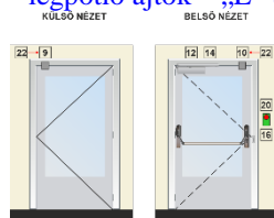
G21. ábra: Egyszárnyú, elektromos zárral rendelkező homlokzati ajtók / tűzgátló vagy lépgátló ajtók – „E” típus
