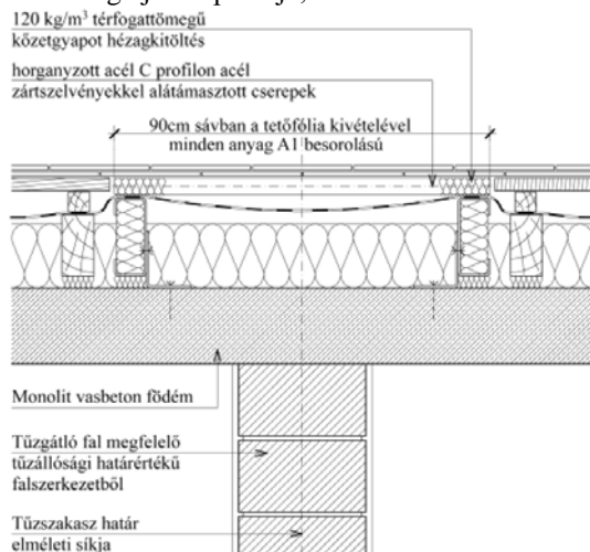
F4 sz. ábra: magastető tetősíkból tartott tetőszinti tűzterjedés elleni gátja kialakításának példája, vasbeton koporsófödém esetén
