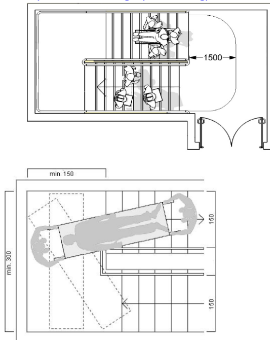
14. ábra: 2Kerekessel és hordágyal történő mentésre alkalmas lépcsőház minimális méretei
