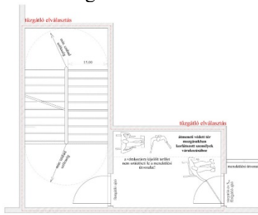
F3. ábra Függőleges tűzszakasz-határral szintenként két tűzszakaszra osztott épületrész, két átmeneti védett tér és lépcsőház együttesével, mindkét oldalon menekülési felvonóval
