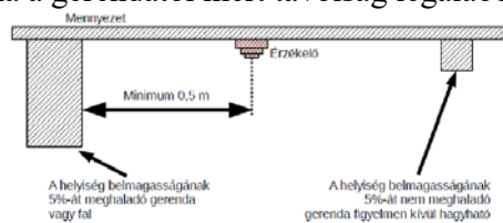
3. ábra Füstérzékelő távolsága gerendáktól
