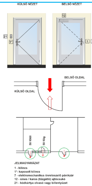
G18. ábra: Egyszárnyú, elektromos zárassal rendelkező homlokzati ajtók / tűzgátló ajtók – „B” típus
