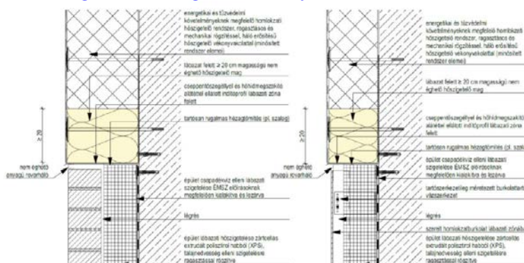
M3 ábra Csomópont javasolt elvi kialakítása légrésez lábazatok esetében
