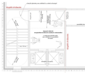
F3. ábra Függőleges tűzszakasz-határral szintenként két tűzszakaszra osztott épületrész, két átmeneti védett tér és lépcsőház együttesével, mindkét oldalon menekülési felvonóval
