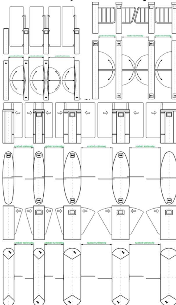
C8. ábra: Ajtók szabad szélessége
