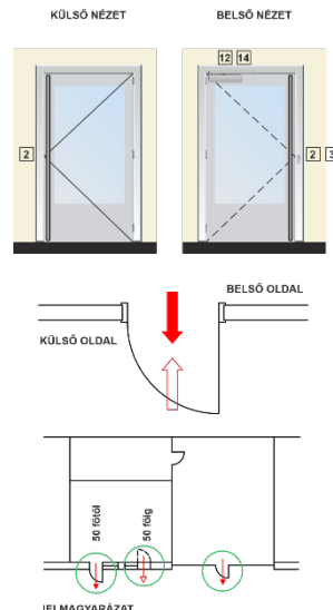
G10. ábra: Egyszárnyú, elektromos zárassal rendelkező belső ajtók / tűzgátló ajtók – „D” típus
