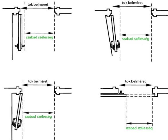
C8. ábra: Ajtók szabad szélessége
