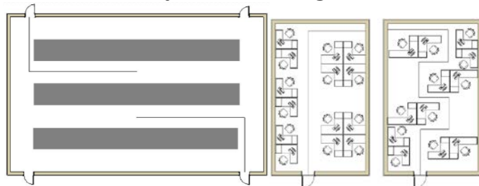
C1. ábra: Példák a kiürítési út hosszának megállapítására
