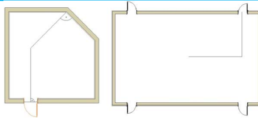
C2. ábra: Példák a kiürítési út hosszának megállapítására
