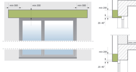
7.5.2. ZABEZPIECZENIE OKNA OSADZONEGO W WARSTWIE IZOLACJI
